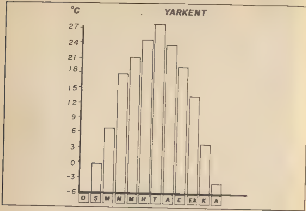
Şekil 4 - Yarkent'in sıcaklık rejimi
